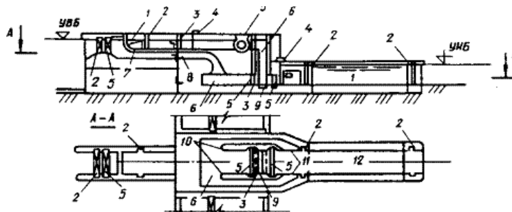
Черт.5. Рыбодъемные сооружения. Гидравлический рыбодъемник
